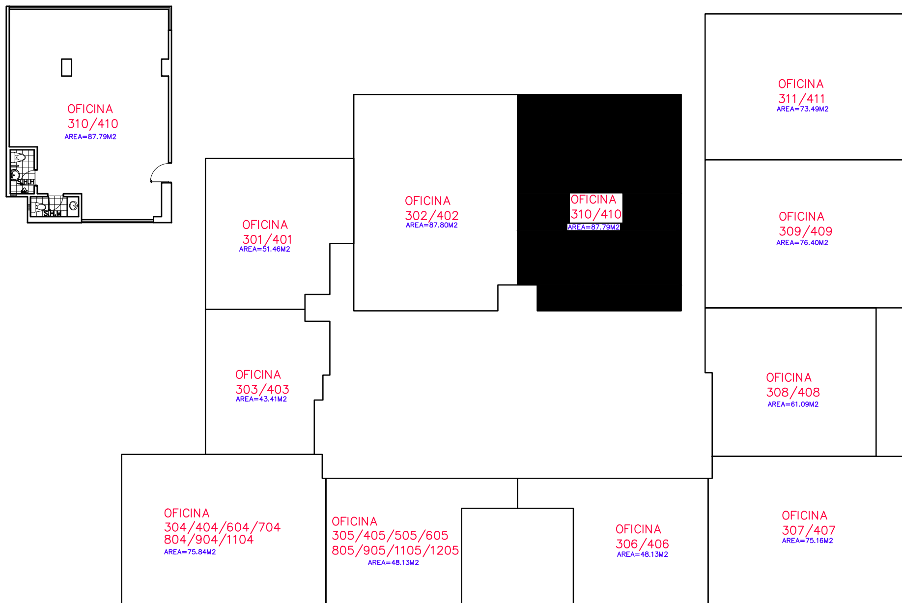
PLANTA 3°,4°,5°,6°,8°,9°,11°,12° PISO
